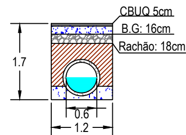
Detalhe escavação Tubo Ø600 s/b
