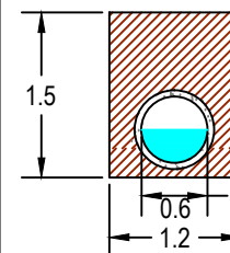
Detalhe escavação Tubo Ø600 s/b
