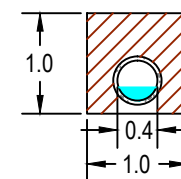
Detalhe escavação Tubo Ø400 s/b
