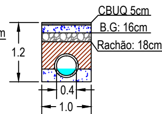
Detalhe escavação Tubo Ø400 c/b
